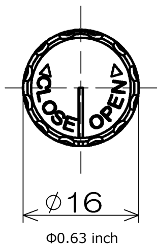
■ Knob Dimensions
